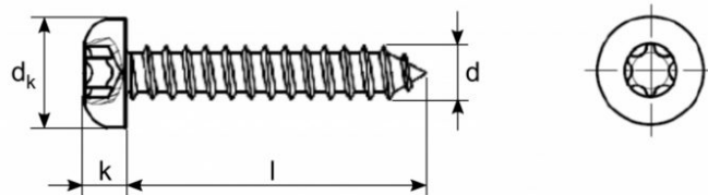
Wymiary Dimensions
