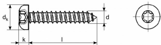
Wymiary Dimensions
