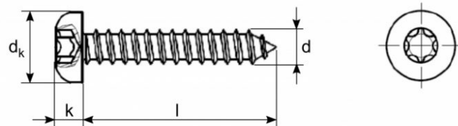
Wymiary Dimensions
