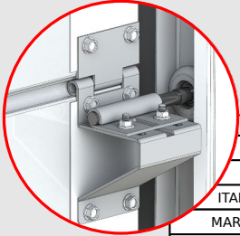
SIDE HINGE
